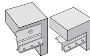
A parete/soffitto
