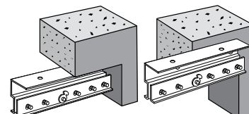
A parete/soffitto
