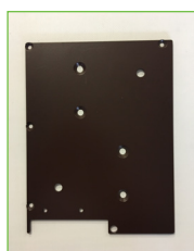
TESTATA LATERALE DUO' Duo' side head Endkappe für Duo' Tête latérale pour caisson Duo'
